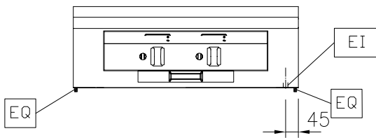
Alzado
